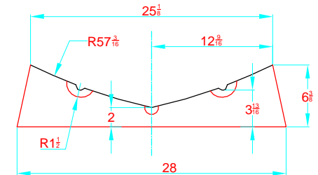
TRANSVERSAL SECTION "B" SECCION TRANSVERSAL "B"
